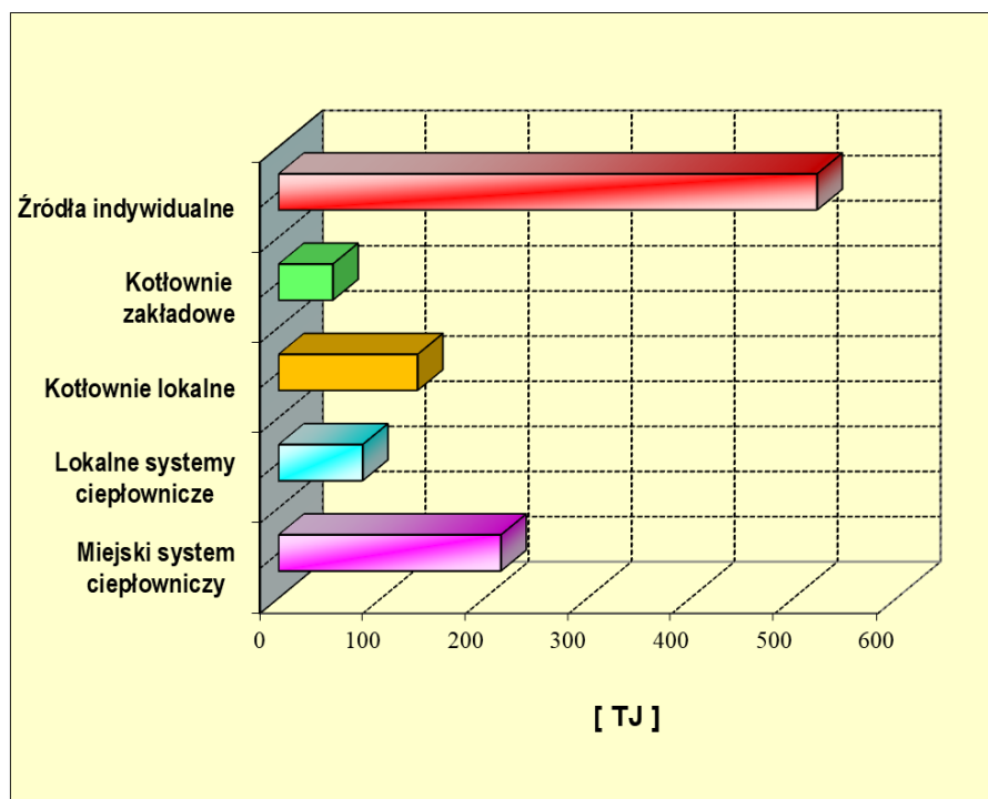
Rys. 1.3 Aktualna struktura zapotrzebowania na energię ciepłą odbiorców na terenie miasta Chojnice [Tj]
