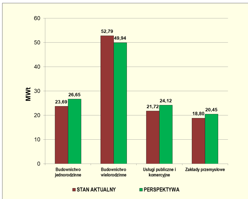
Rys. 4.4.3. Aktualne i perspektywiczne zapotrzebowanie na moc ciepłą poszczególnych grup odbiorców na obszarze miasta Chojnice [MW]
