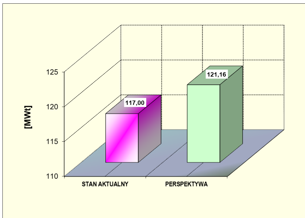
Rys. 4.4.1. Aktualne i perspektywiczne zapotrzebowanie na moc cieplną na obszarze miasta Chojnice [MW]
